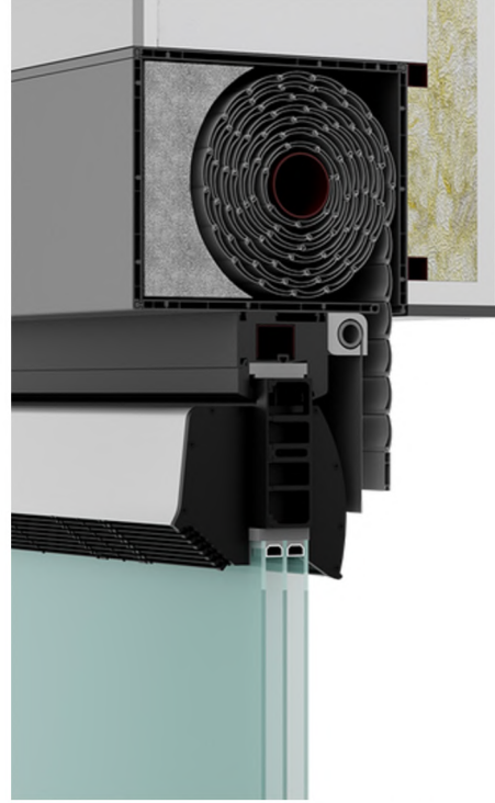
Doğrama İçi Yatay Sercair - Monoblok Panjur Montajı Detayı - Perspektif
