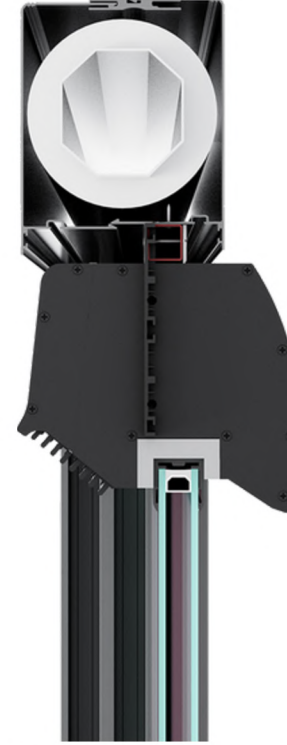
Giyotin Profili-Çift Cam-S1 Kesit
