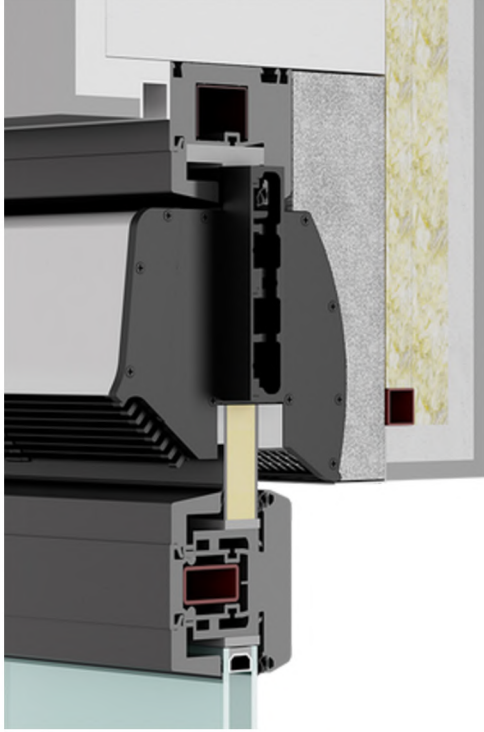
Yatay Sercair - Üst Sabit Doğrama İçi (Orta Kayıt) - Perspektif
