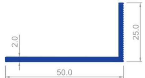
1642 0,388 Kg/m
