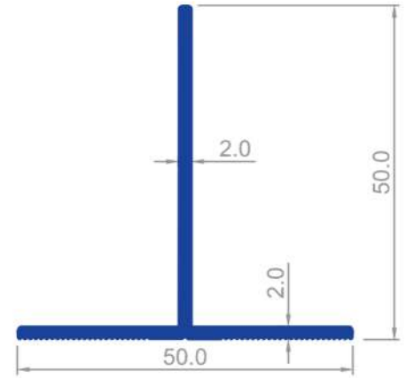
1622 0,518 Kg/m
