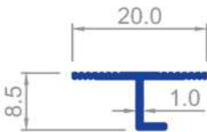
1606 0,080 Kg/m
