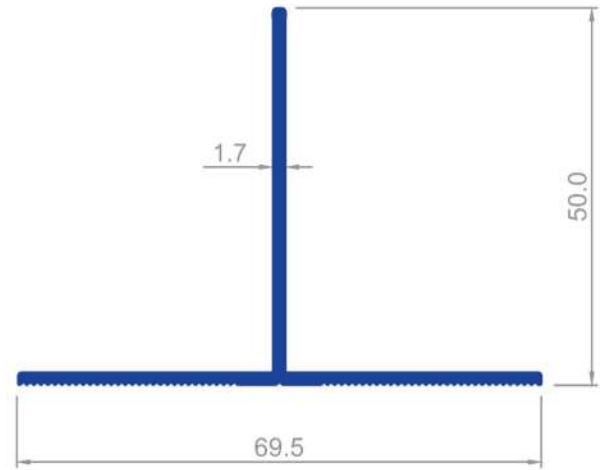
1600 0,523 Kg/m
