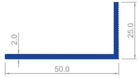
1642 0,388 Kg/m
