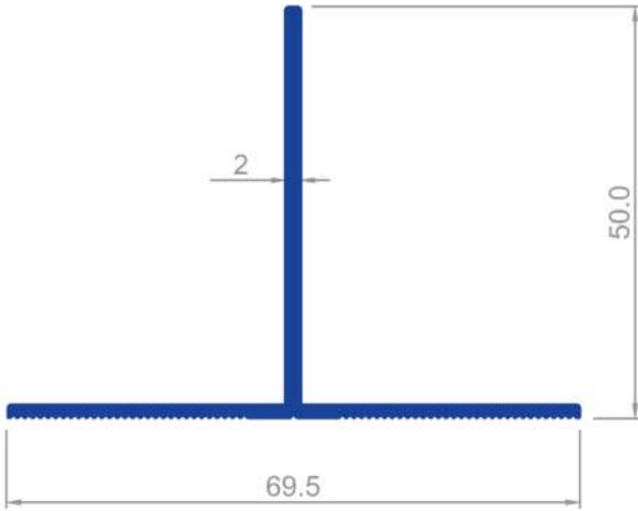
1626 0,618 Kg/m
