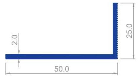
1642 0,388 Kg/m
