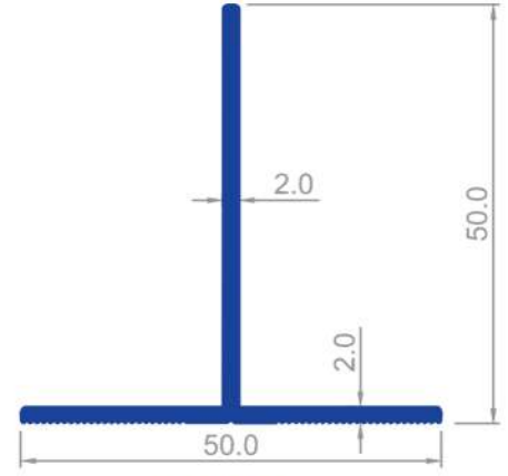
1622 0,518 Kg/m
