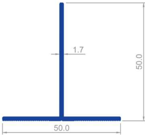
1621 0,439 Kg/m
