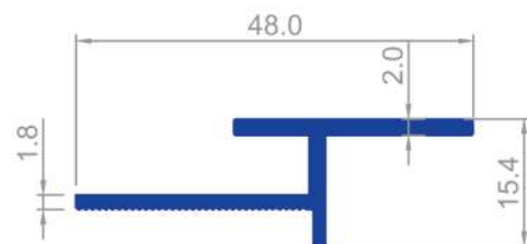
1653 0,352 Kg/m
