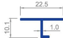
1607 0,095 Kg/m
