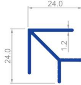
1613 0,246 Kg/m
