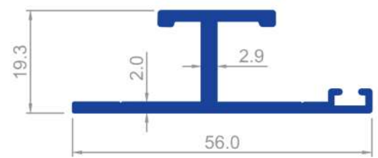
1654 0,567 Kg/m
