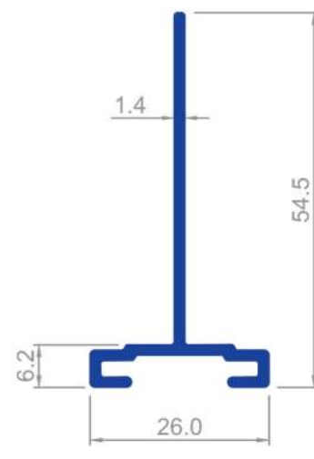
1618 0,350 Kg/m
