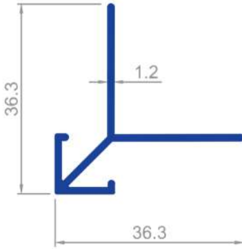
1610 0,285 Kg/m
