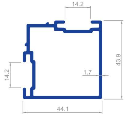
1609 0,875 Kg/m
