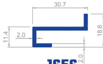
1656 0,295 Kg/m
