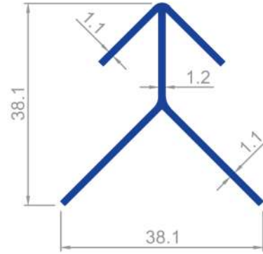
1644 0,309 Kg/m
