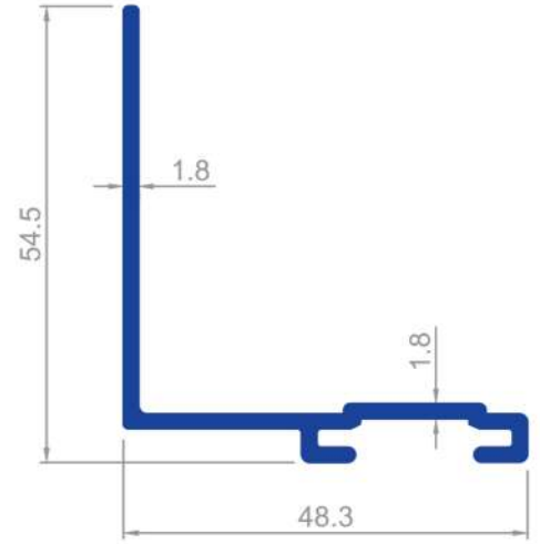
1604 0,565 Kg/m
