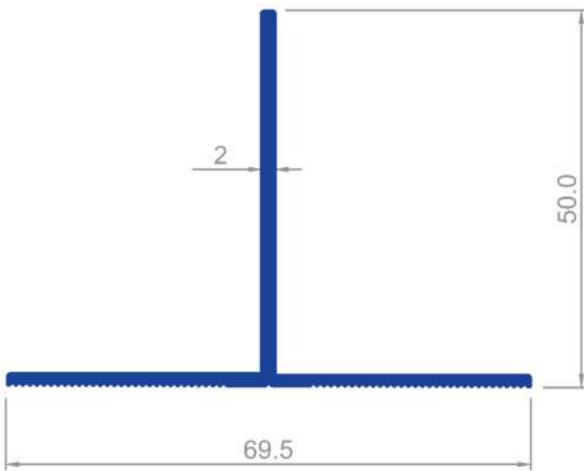
1626 0,618 Kg/m
