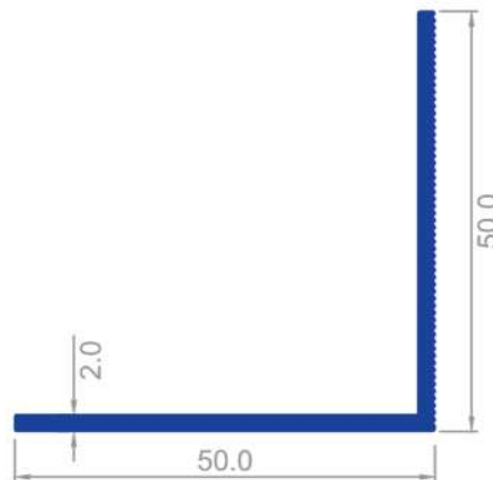
1641 0,516 Kg/m
