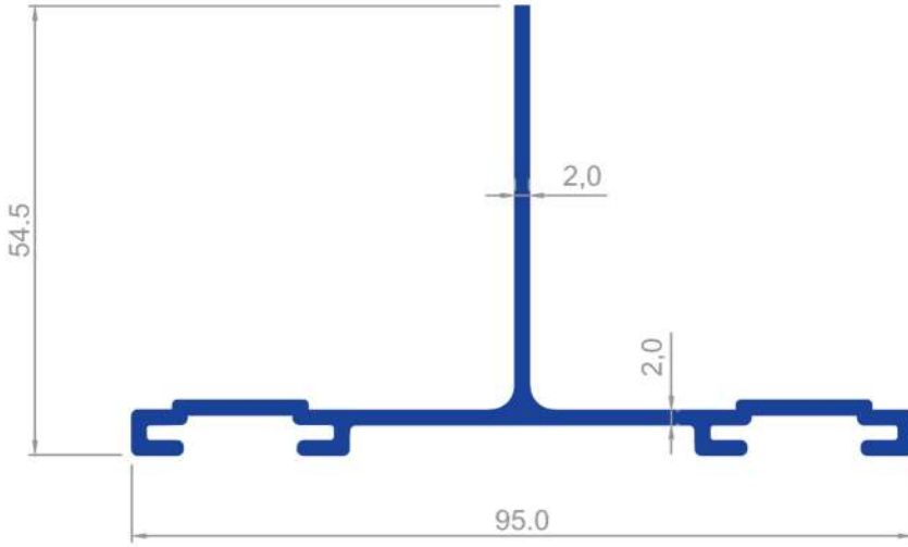
1602 0,995 Kg/m
