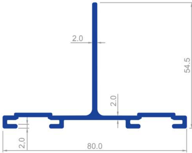
1601 0,905 Kg/m
