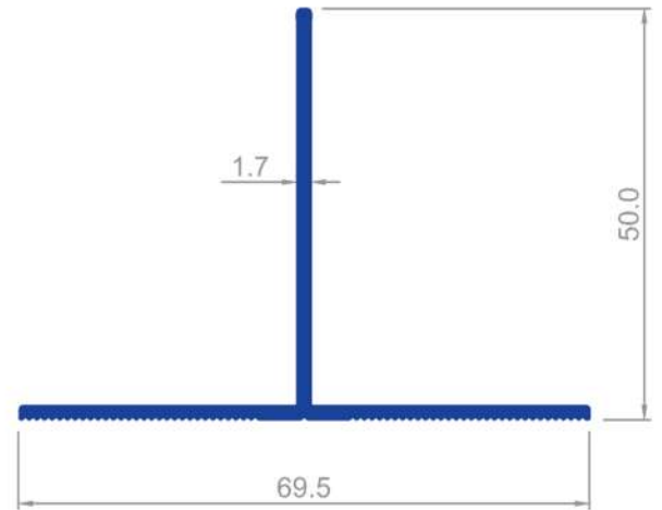
1600 0,523 Kg/m
