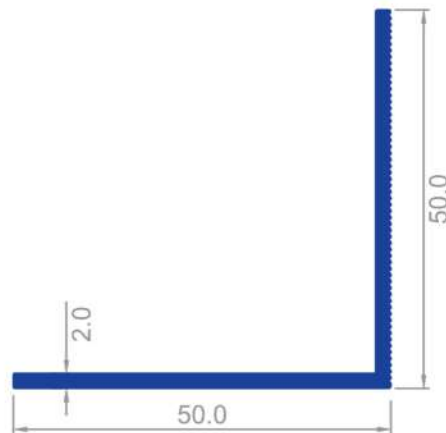
1641 0,516 Kg/m
