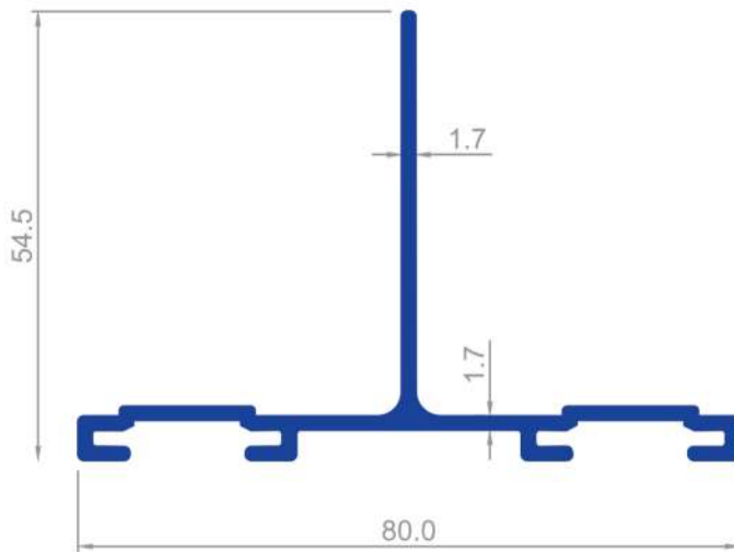
1616 0,771 Kg/m
