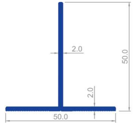
1622 0,518 Kg/m
