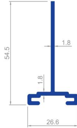
1603 0,452 Kg/m
