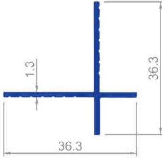
1643 0,246 Kg/m
